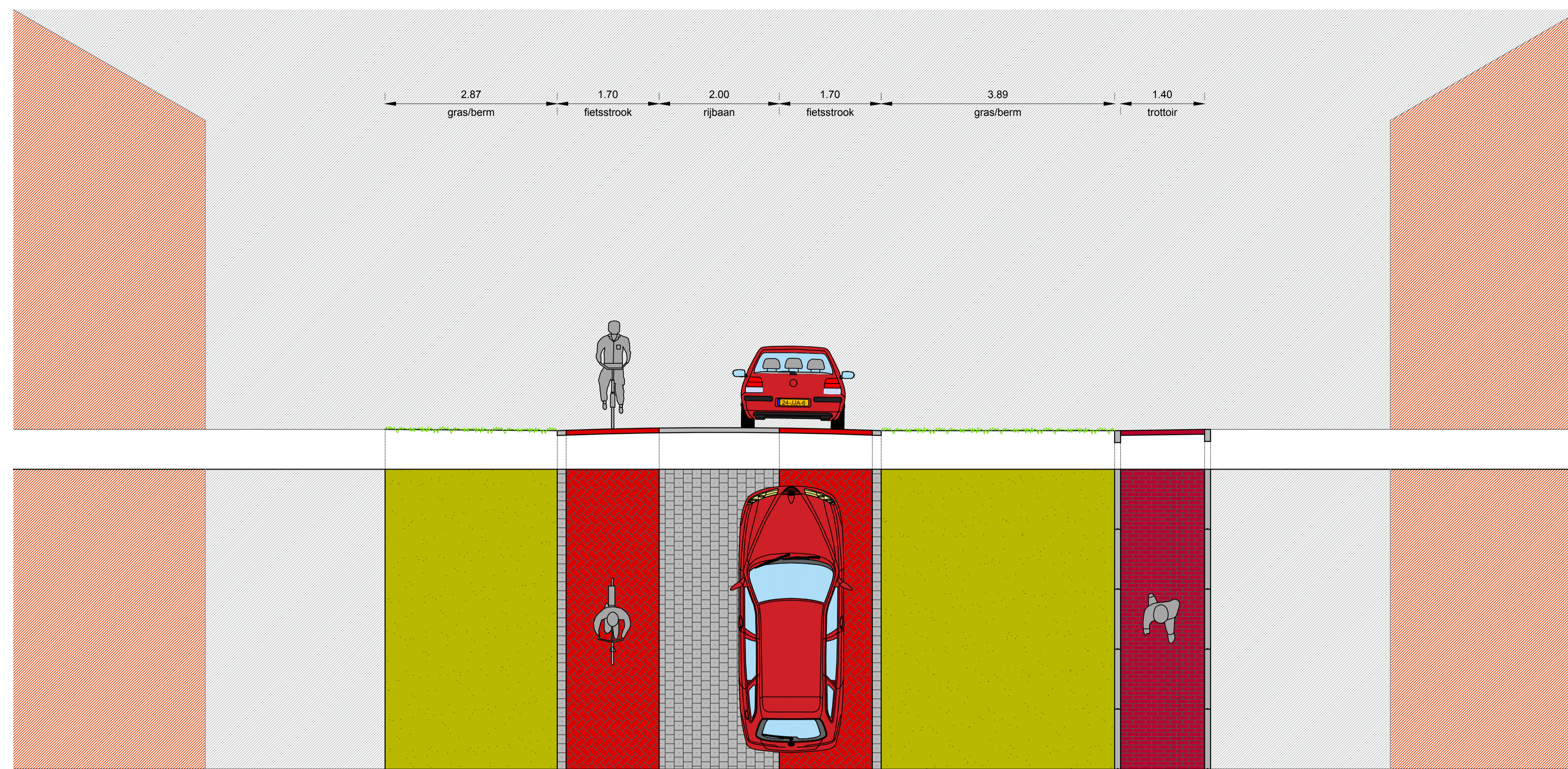
Dwarsprofiel A-A schaal: 1 : 50
