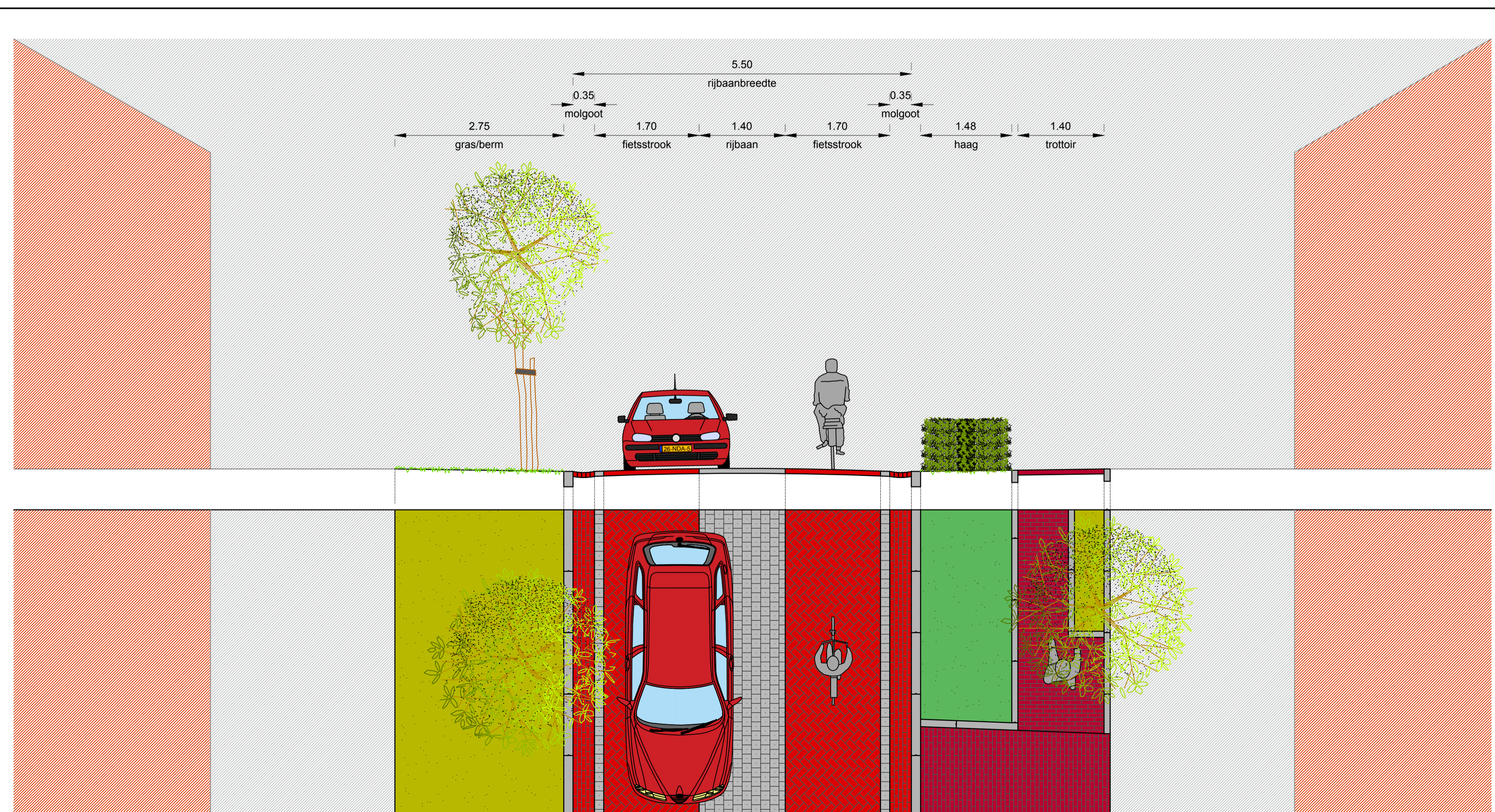
Dwarsprofiel B-B schaal: 1 : 50
